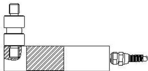
NB2 型传感器用球座 Tee for NB2 type load cell
